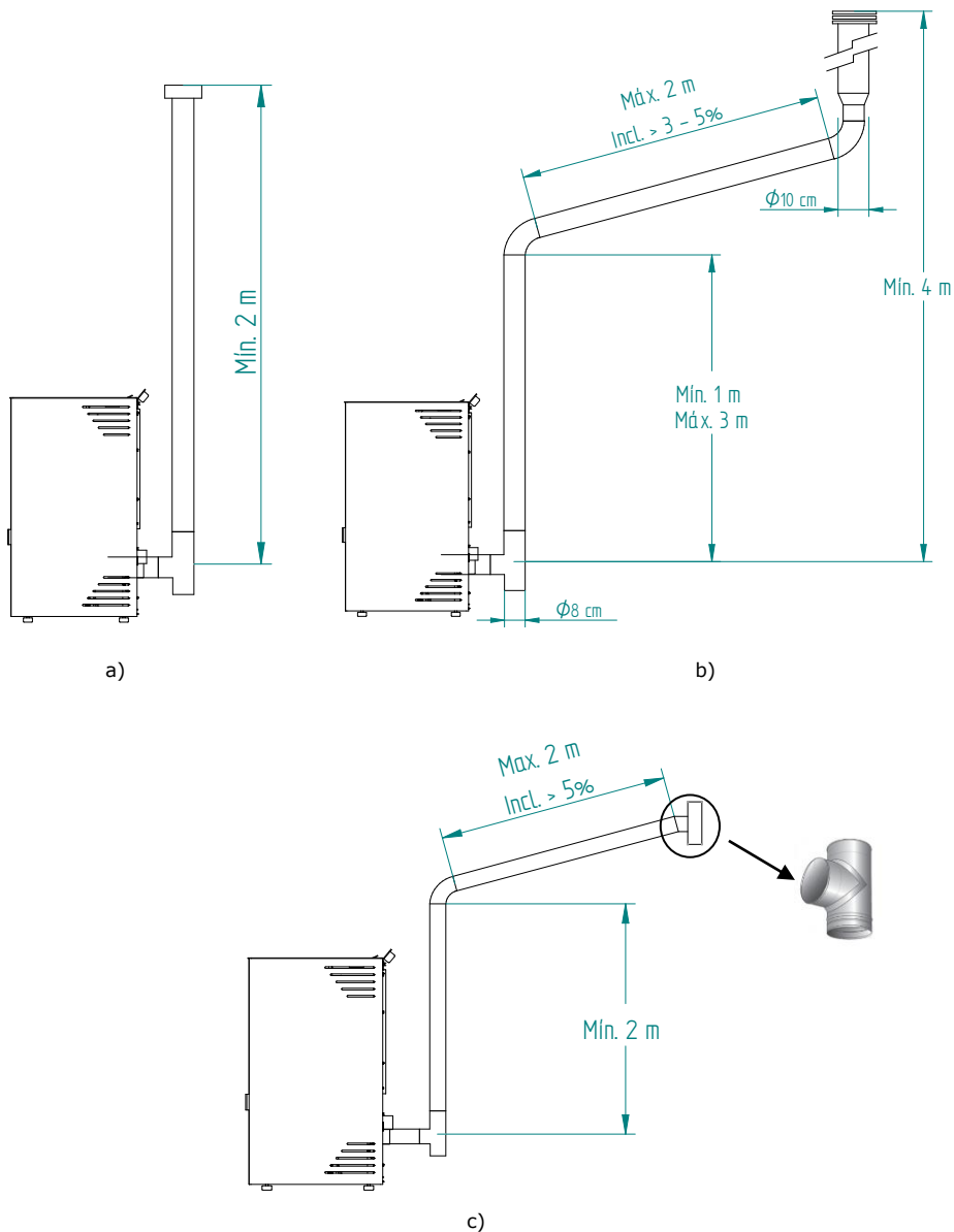
Figura 6 – Exemplos de instalações tipo
