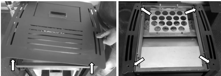
Figura 15 - Remoção tampo superior
