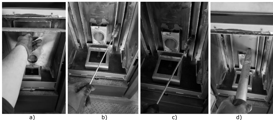
Figura 24 - Limpeza câmara de combustão
