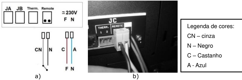
Figura 31 - Ligação do comando remoto sem fios
