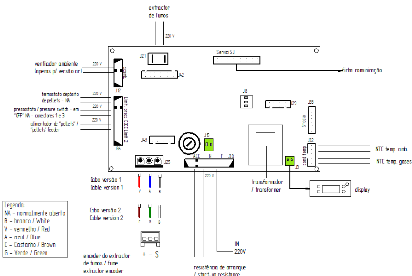
Figura 60 - Esquema elétrico
